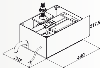
Dimensioni (mm)
