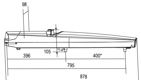
DIMENSIONS (mm) * with mechanical stops corsa con battute meccaniche montate
