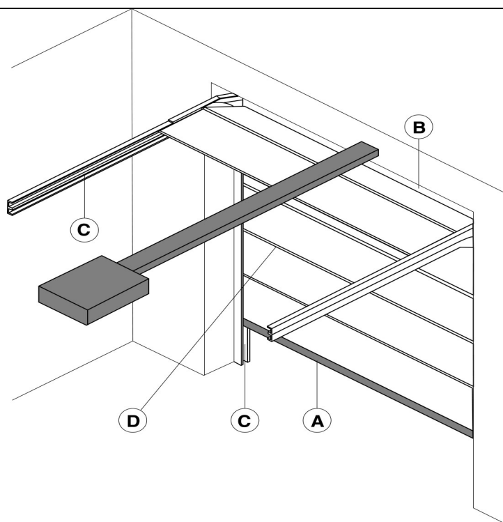
Zone di rischio della porta sezionali da garage (figura 1)
