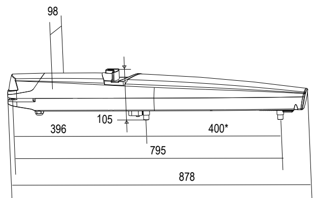
DIMENSIONI (mm)
